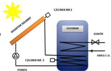
3. Ładowanie zasobnika C.W.U. przez kolektor solarny oraz kocioł C.O. dwie węzownice
